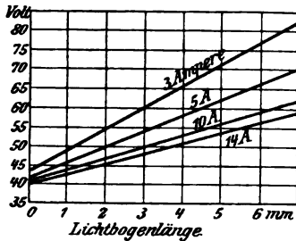
Abb. 367. Lichtbogenlänge zwischen Kohlenelektroden.
